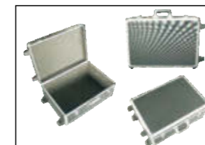
ITEM:APC019 Material:AL,ABS I D:L570×W395×H240 mm OD:L580×W405×H250 mm
